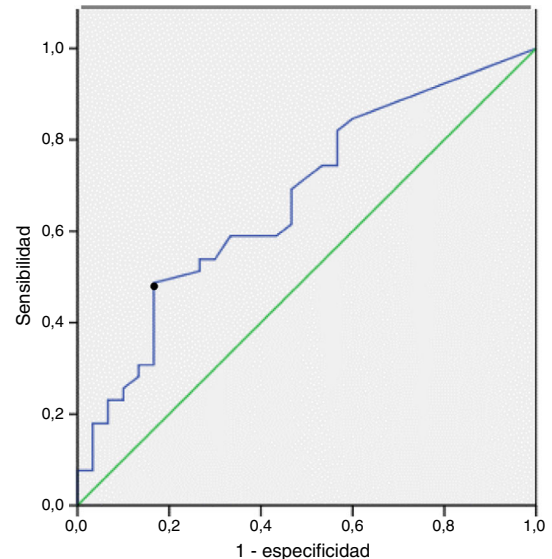
Figura 2. Curva de características operativas del receptor construida para determinar el valor más relevante de CA/ml de LBA para la predicción de ERA. El punto indica el valor de corte óptimo.
