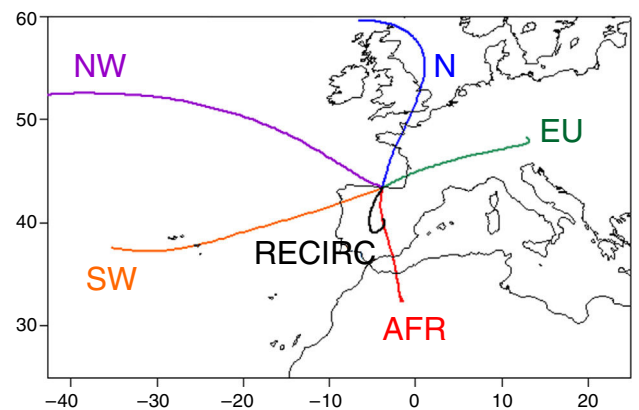
Figura 3. Tipología de las retrotraectorias y origen. AFR: Norte de África y zona mediterránea de la península; EU: Cantábrico francés; N: Islas Británicas; NW Noratlántico; RECIRC: recirculación a nivel peninsular; SW: Sudatlántico portugués.
