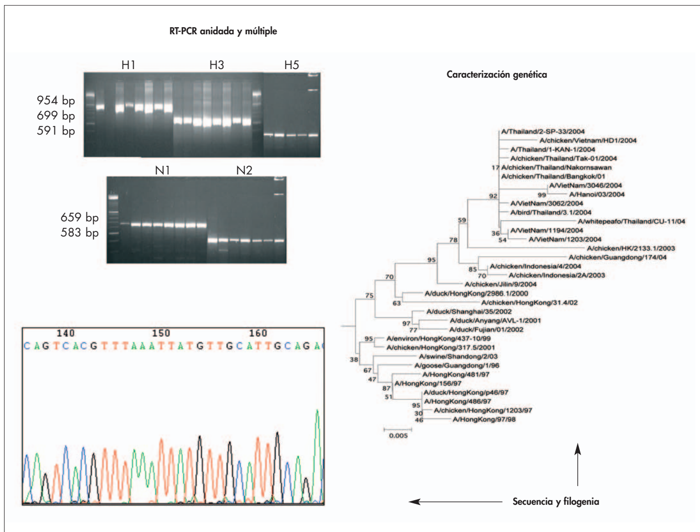
Figura 3. Amplificación genómica por RT-PCR anidada que permite detectar y diferenciar distintas hemaglutininas (H1, H3 y H5) y neuraminidasas (N1 y N2) de virus gripales del género Influenza A. Hoja de lectura de la secuencia de un fragmento amplificado y árbol filogenético obtenido al realizar el análisis de ésta, en comparación con otras secuencias de virus gripales de referencia.
